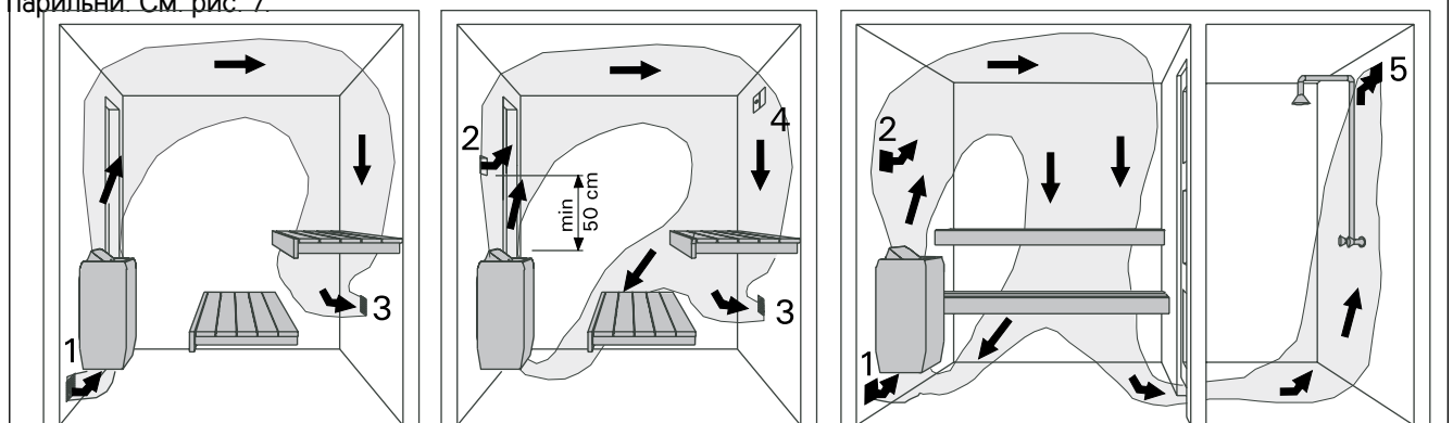
Рисунок 7. Вентиляция в сауне Joonis 7 Leiliruumi ventilatsioon
