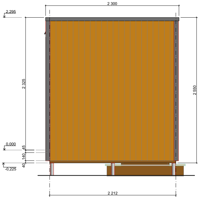
Фасад в осях 2-1
