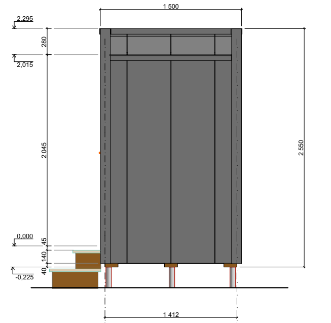
Фасад в осях А-Б
