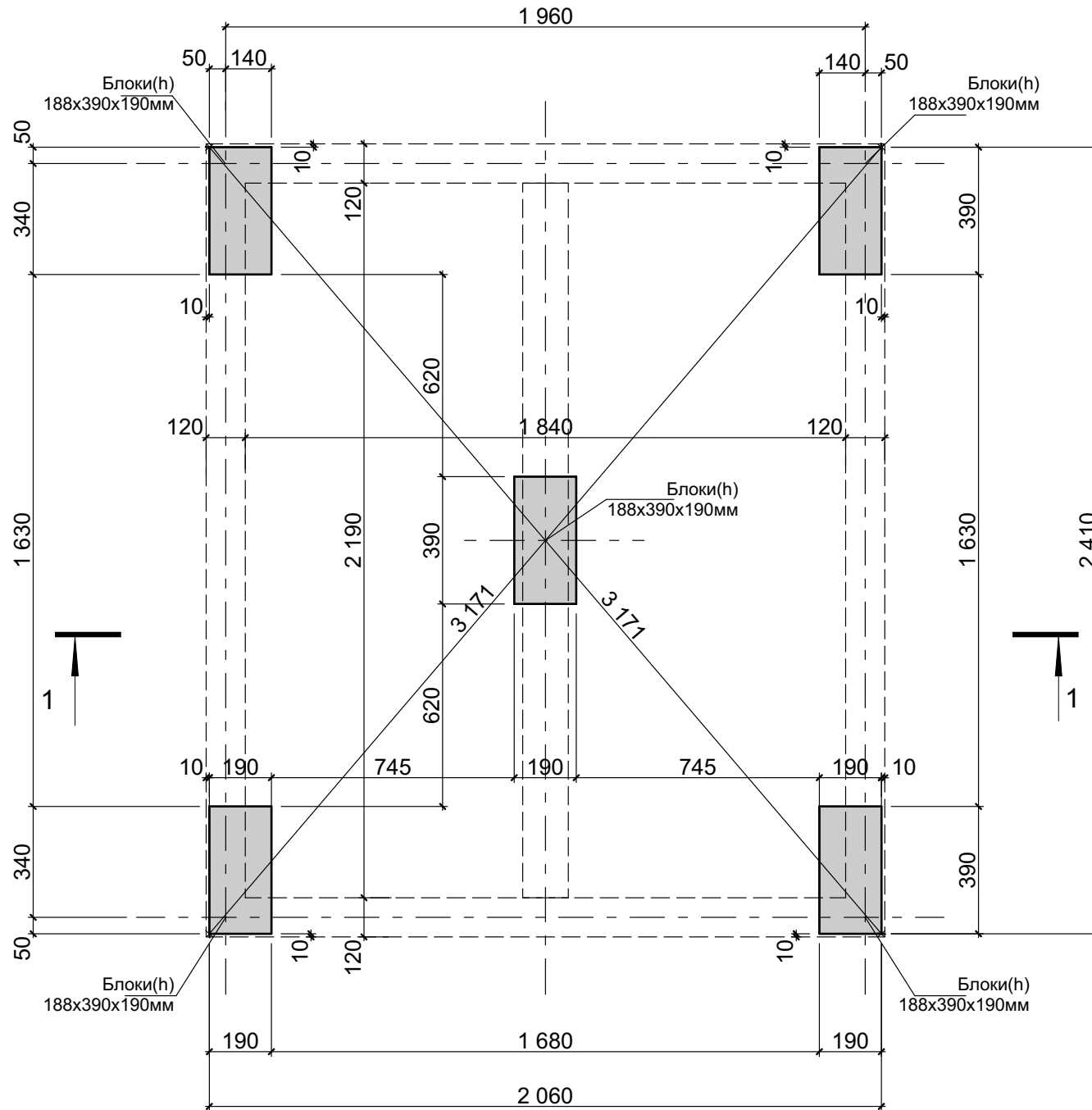
Схема расположения фундаментных блоков для бани габаритом 2,55х2,2м.
